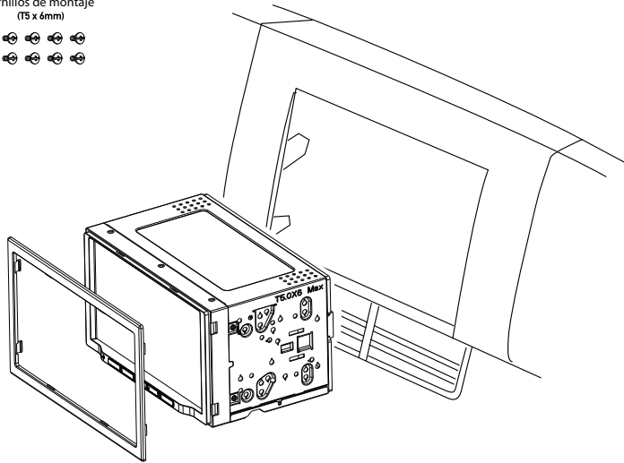
Tornillos de montaje (T5 x 6mm)
